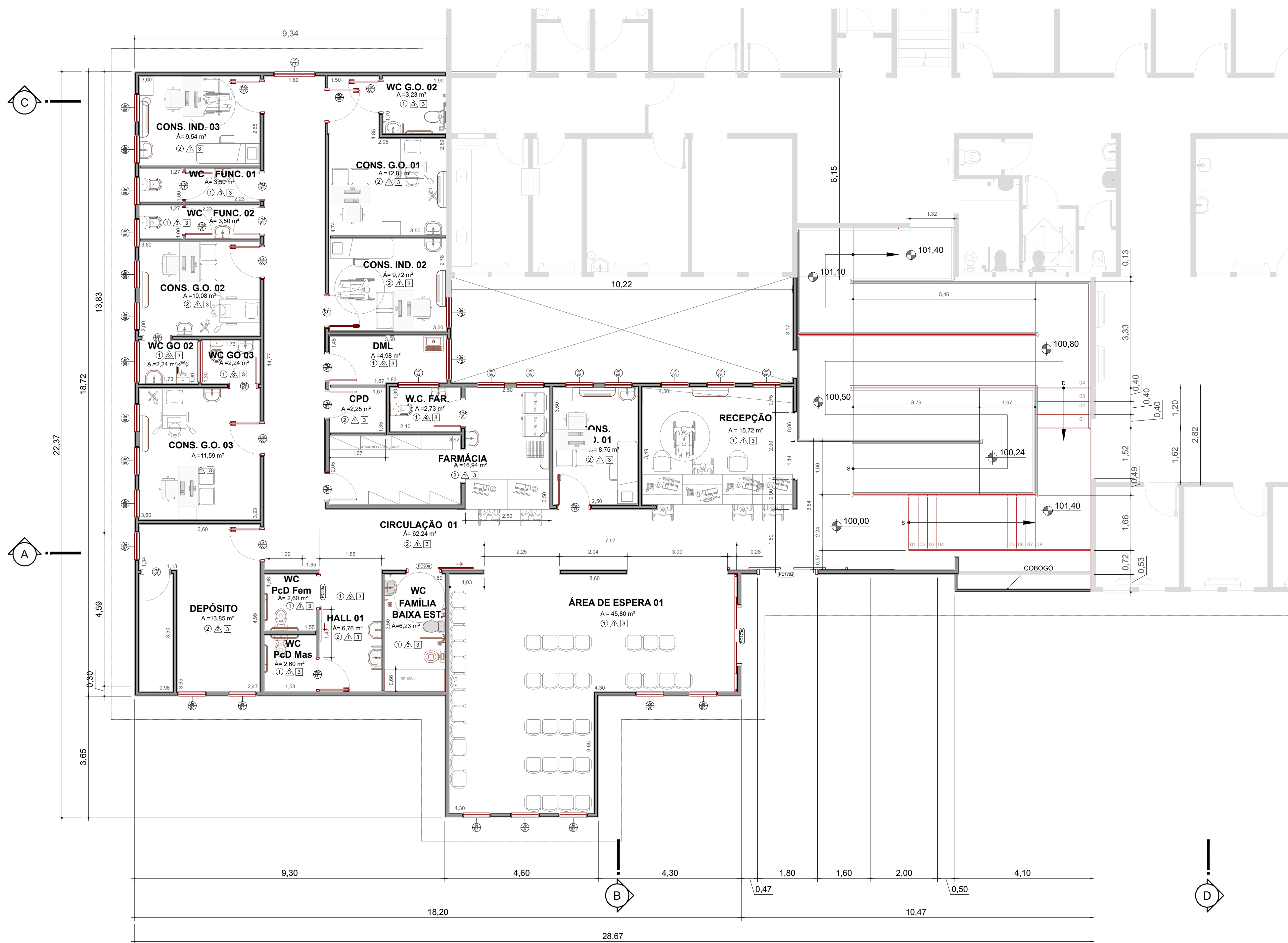
PLANTA DE ARQUITETURA FINAL - PAV. INFERIOR ESC: 1:100
