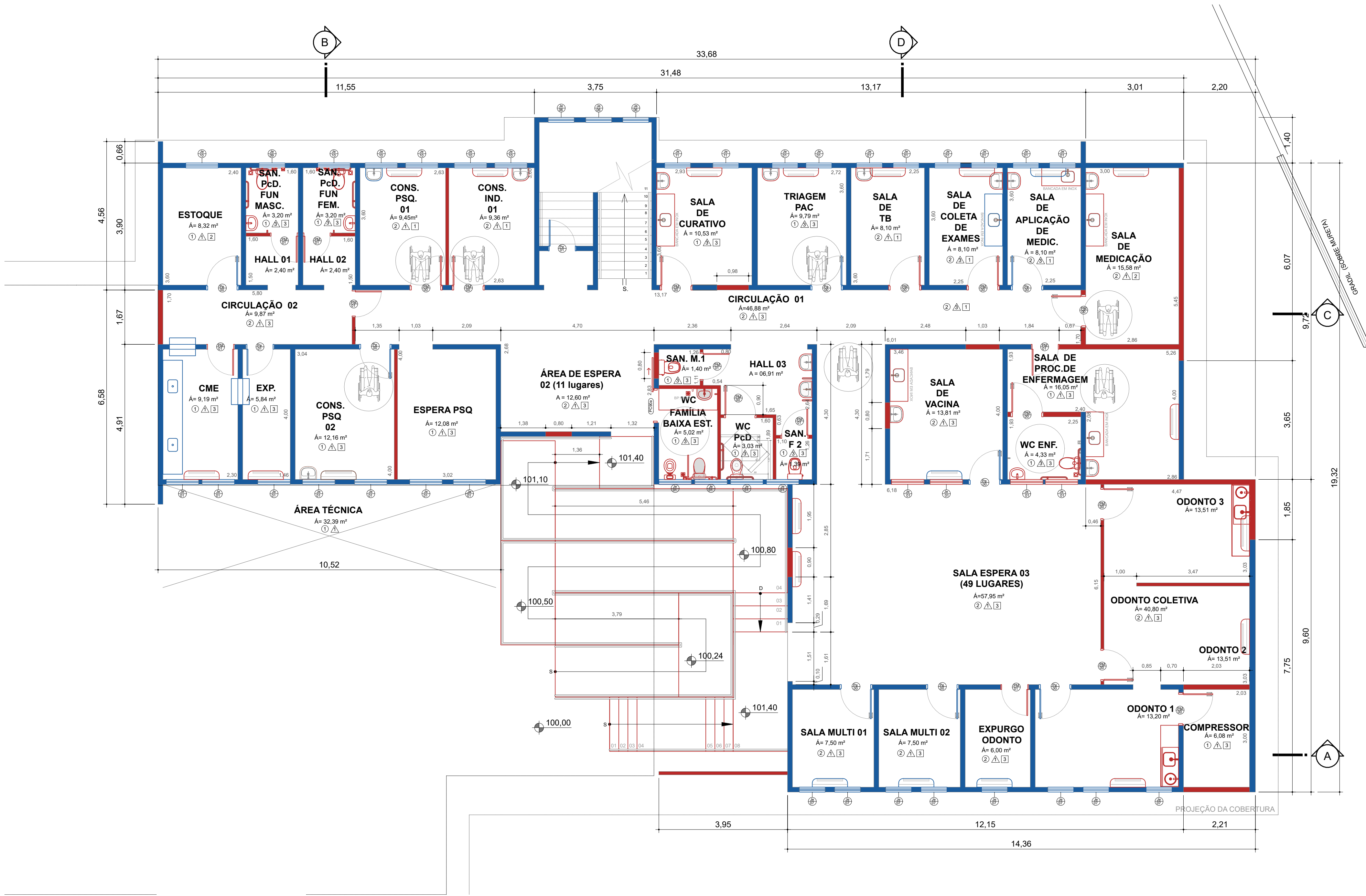
PLANTA DE ARQUITETURA FINAL - PAV. INTERMEDIÁRIO ESC: 1:100
